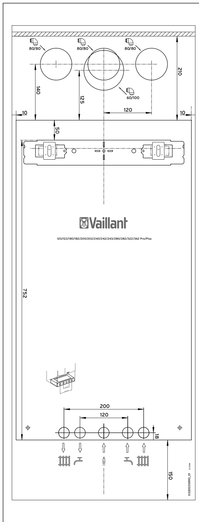
Мал. 4.4 Монтажный шаблон
