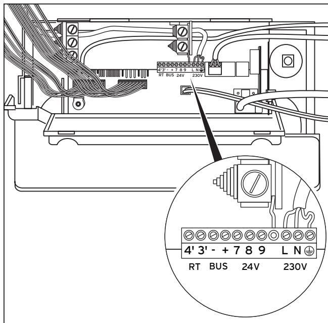
Мал. 5.13 Приклад прокладки кабелів
