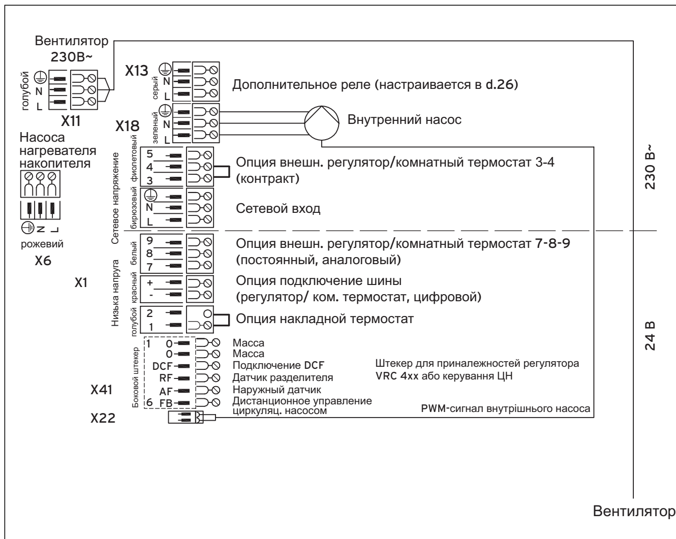
Мал. 5.14 Схема підключення ecoTEC plus (продовження)
