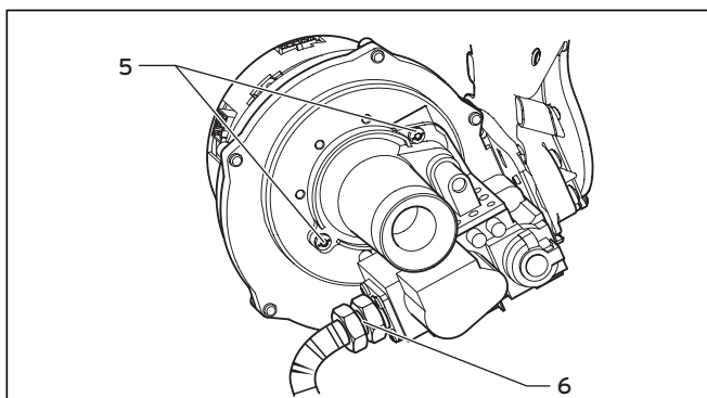
Мал. 10.3 Різьбове з'єднання газова арматура/вентилятор
