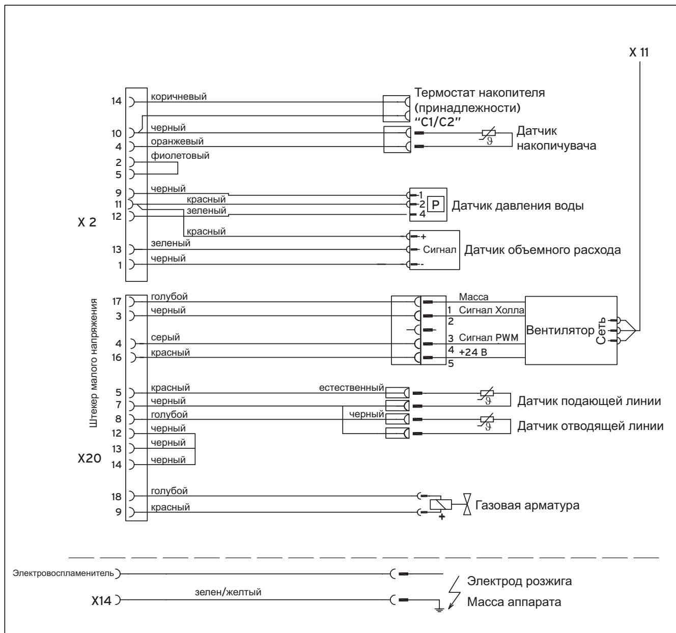
Мал. 5.14 Схема підключення ecoTEC plus (продовження на наступній сторінці)
