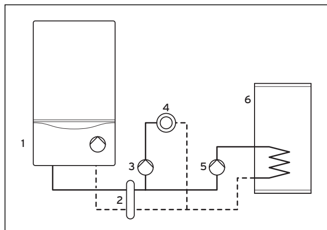
Мал. 5.5 Пріоритетна схема накопичувача та опалювального контуру через гідравлічний чан
