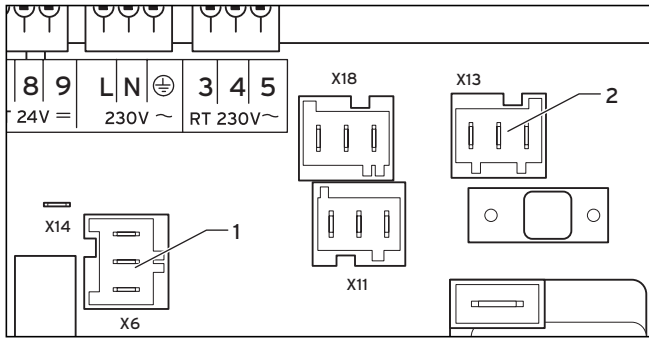
Мал. 5.6 Електропідключення насосу нагрівання накопичувача та зовнішнього насосу системи опалення
