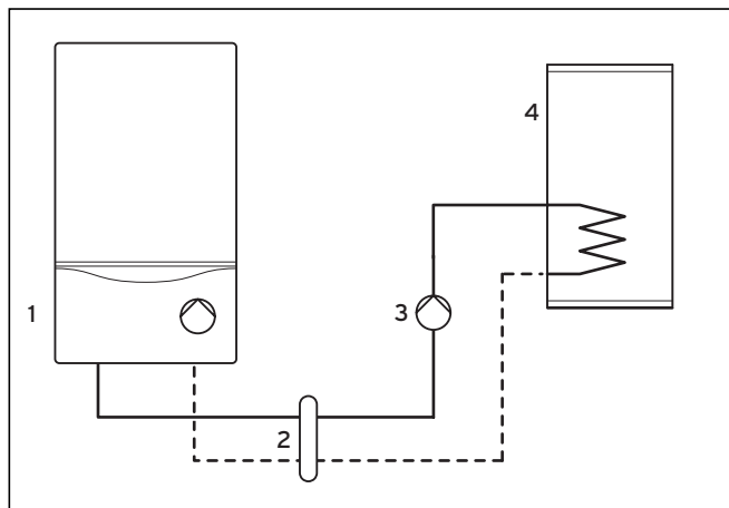
Мал. 5.3 Пріоритетна схема накопичувача через гідравлічний чан
