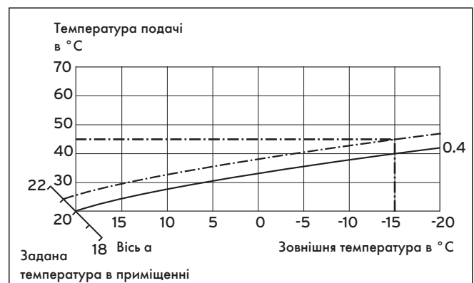
Мал. 2 Паралельне переміщення опалювальної кривої
