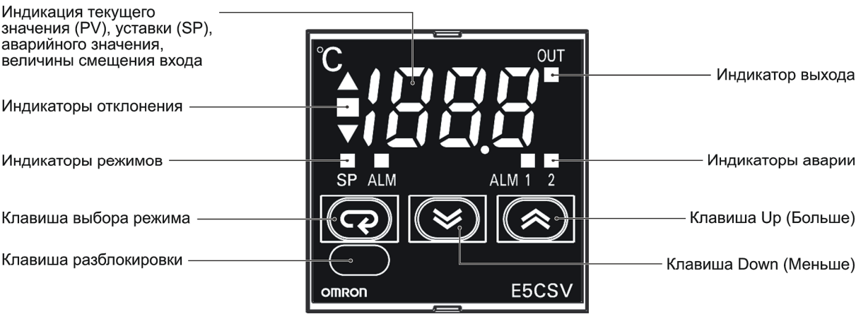
Рис. 2 Регулятор температуры котла
