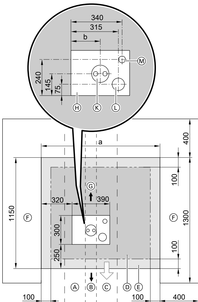
Фундамент - вид сверху
