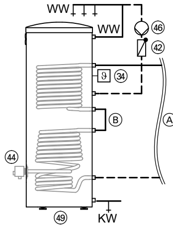
Гидравлическая схема при использовании Vitocell 100-B, тип CVB, 300 л или Vitocell 300-B, тип EVB, 300 л
