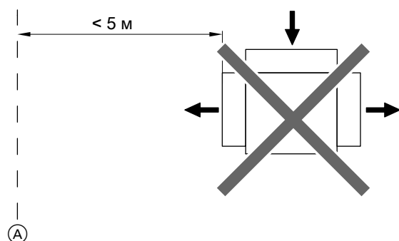
(A) Граница земельного участка
