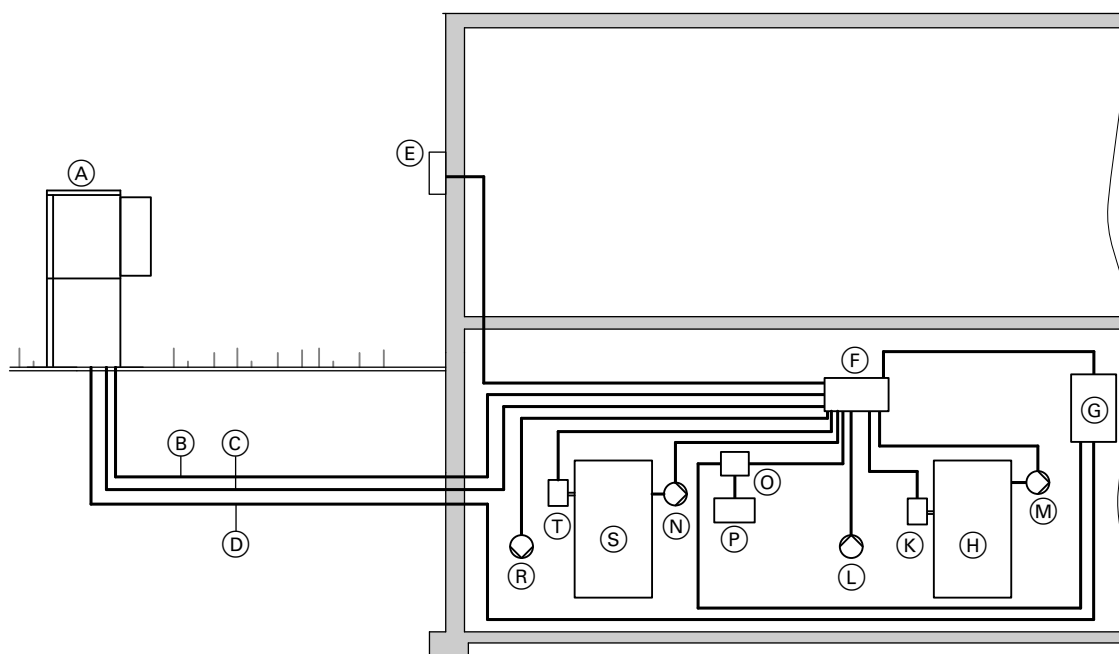
Пример стандартной установки
