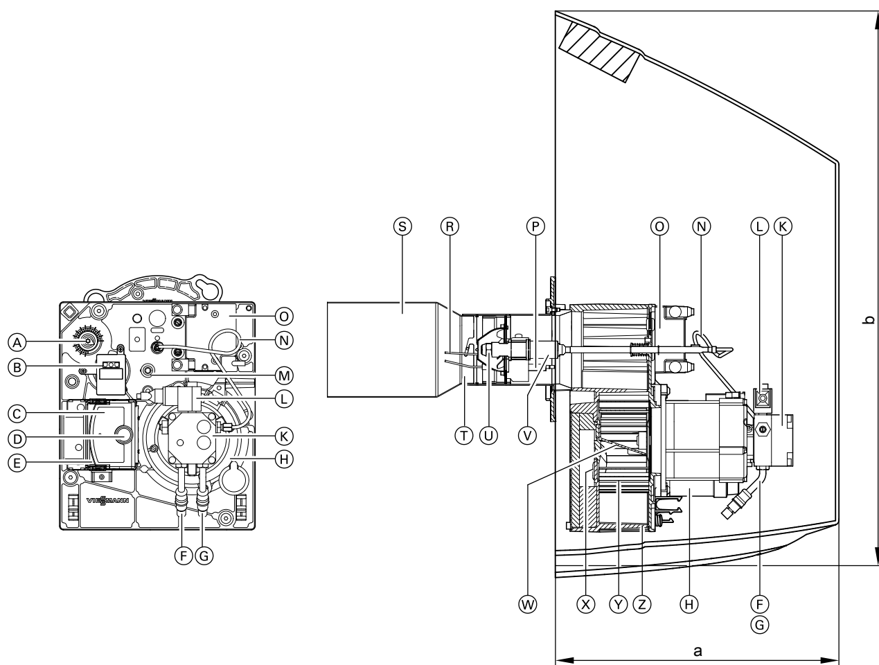
Vitoflame 300, тип VHG мощностью 40 - 50 кВт
