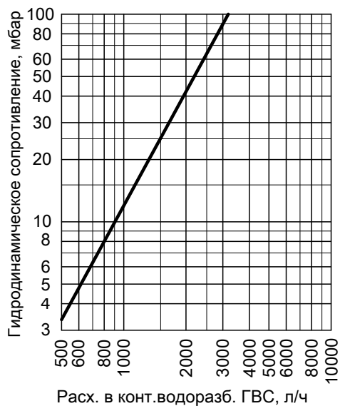
Гидродинамическое сопротивление в контуре ГВС
