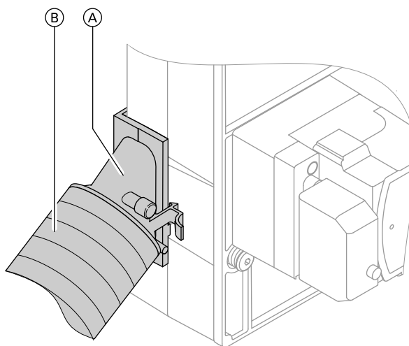
Подключение шланга приточного воздуха (B) с воздухозаборным патрубком (A) в режиме эксплуатации с отбором воздуха для горения извне
