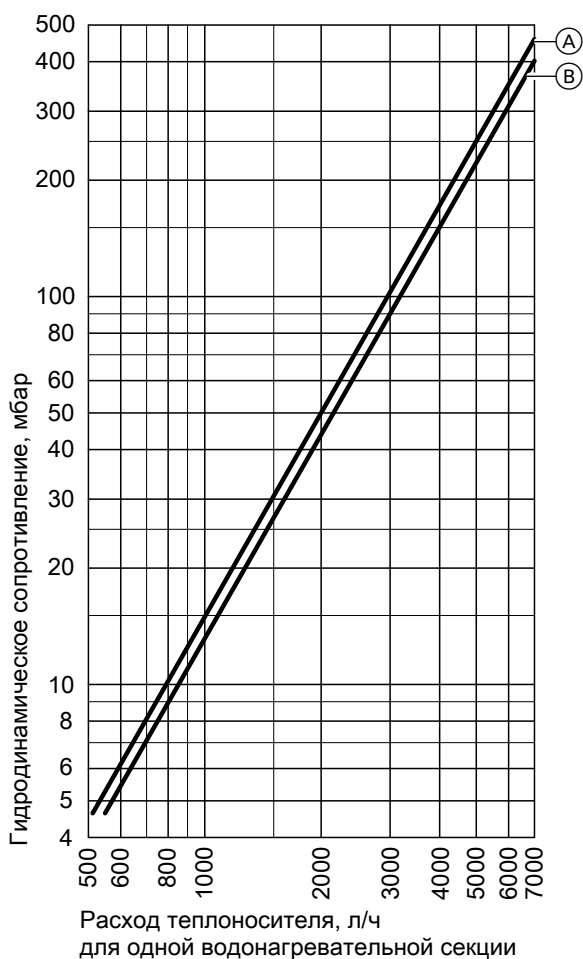
Гидродинамическое сопротивление на стороне греющего контура
