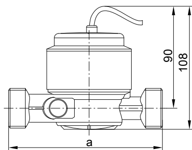
Тепломеры от 06 до 25
