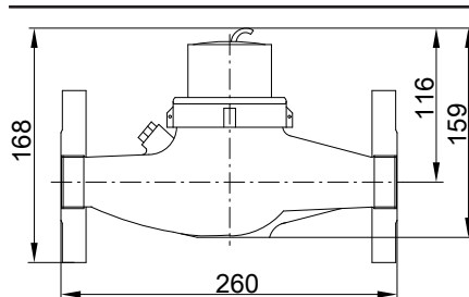
Тепломеры 35 и 60
