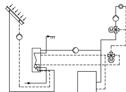
Установка с буферной емкостью Vitocell-M
