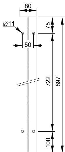
Расположение отверстий опорной стойки
